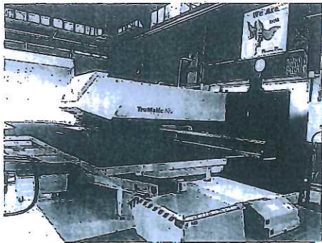
導入したレーザー・パンチング複合機
